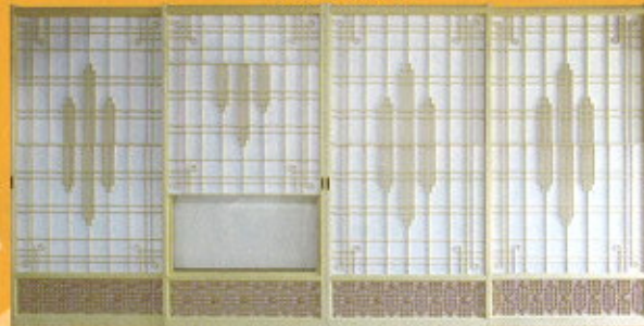
摺り上げ障子(曲げ組子入り)
